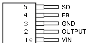
TO-263 5L
