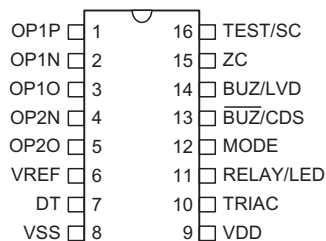
HT7612/HT7612B 16 DIP-A/NSOP-A
