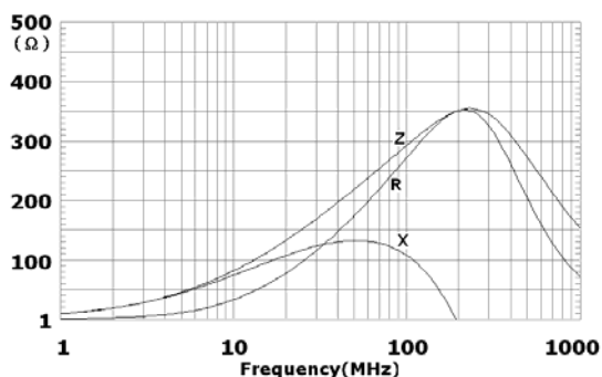
EBMS160808A451
