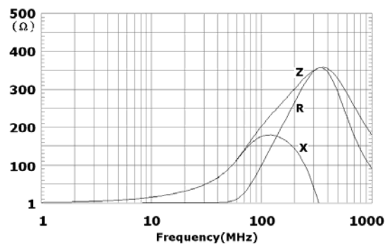
EBMS160808B471
