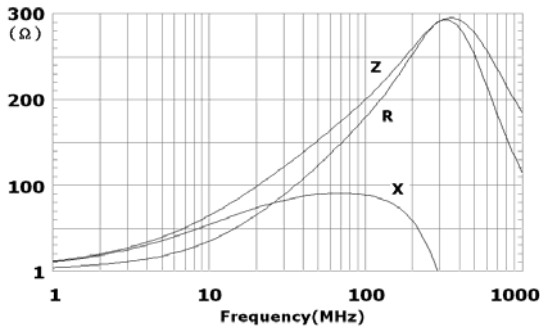
EBMS160808A201
