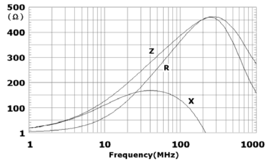
EBMS160808A401
