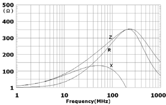
EBMS160808A451
