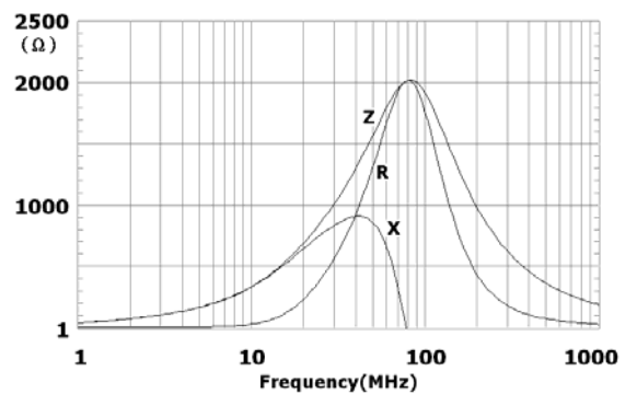
EBMS160808K202
