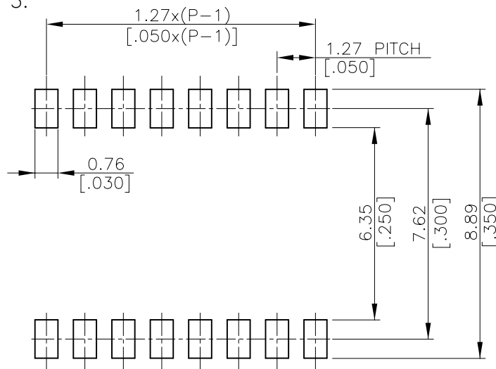
P.C.B LAYOUT
