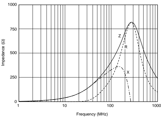
BLM21BD421SN1
