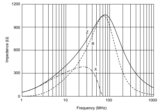
BLM21AH102SN1
